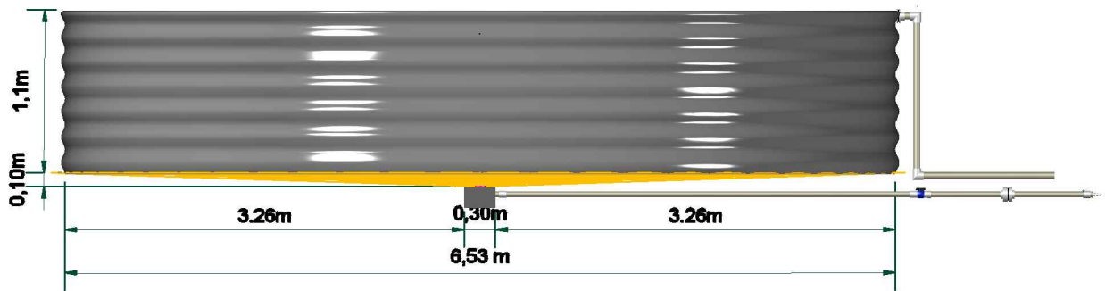
Vista lateral reservoirio Australiano ESCALA 1:35
